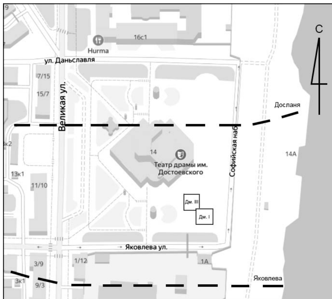
Рис. 1. Ситуационный план раскопов Дмитриевский III (2020) и Дмитриевский I (1976)
