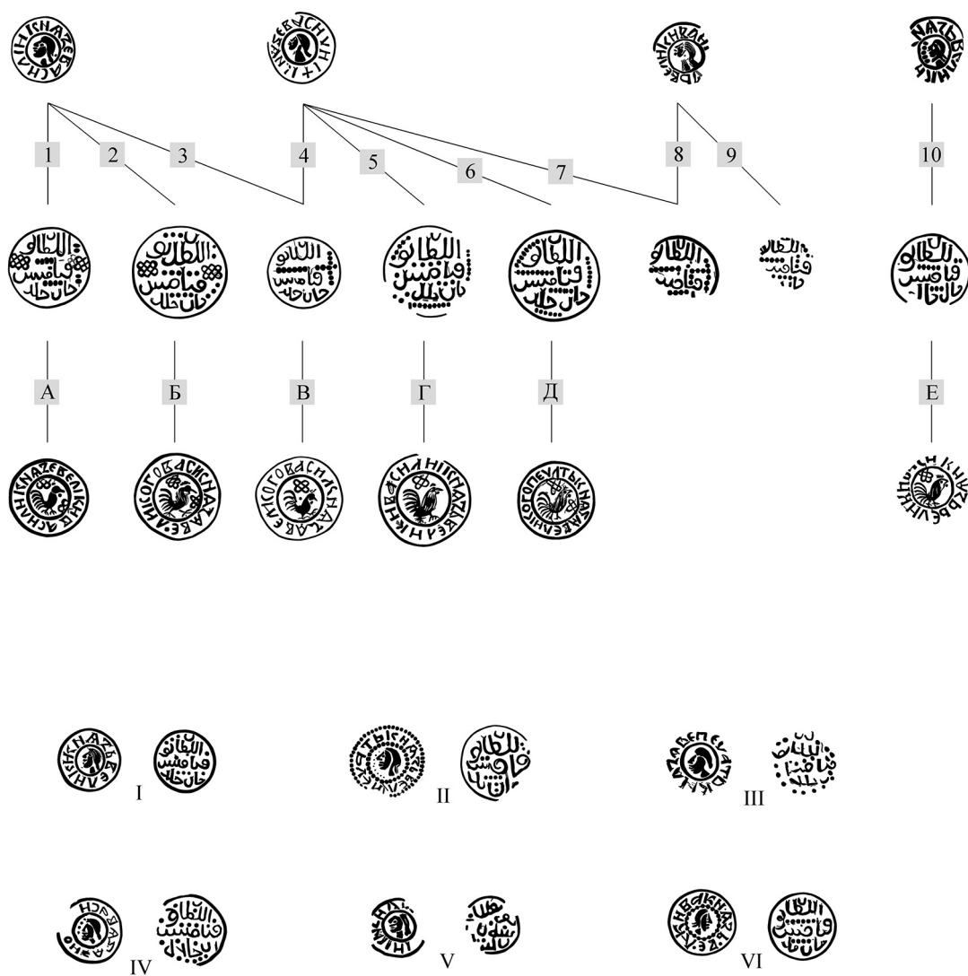
Рис. 1. 1–10 – часть схемы иттемпельных связей полуденег Василия Дмитриевича с изображением головы человека, варианты 1–10; А–Е – варианты денег с изображением петуха, связанные общими иттемпелями оборотных сторон с полуденьями; I–VI – образцы полуденег с изображением головы человека, не вошедших в статью (варианты 11, 16, 18, 20, 27, 14).
